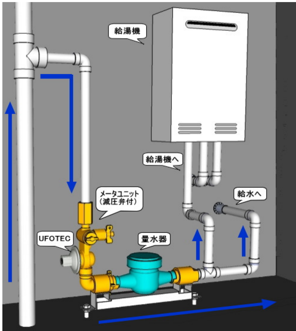
戸別給水集合住宅向けパイプシャフト内の配管設置例
