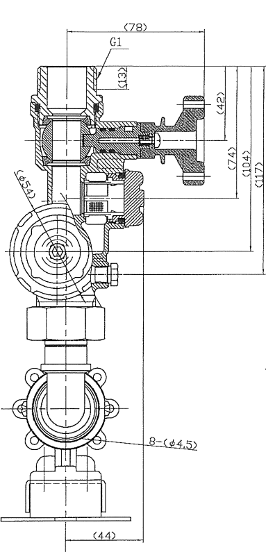
BB断面図
