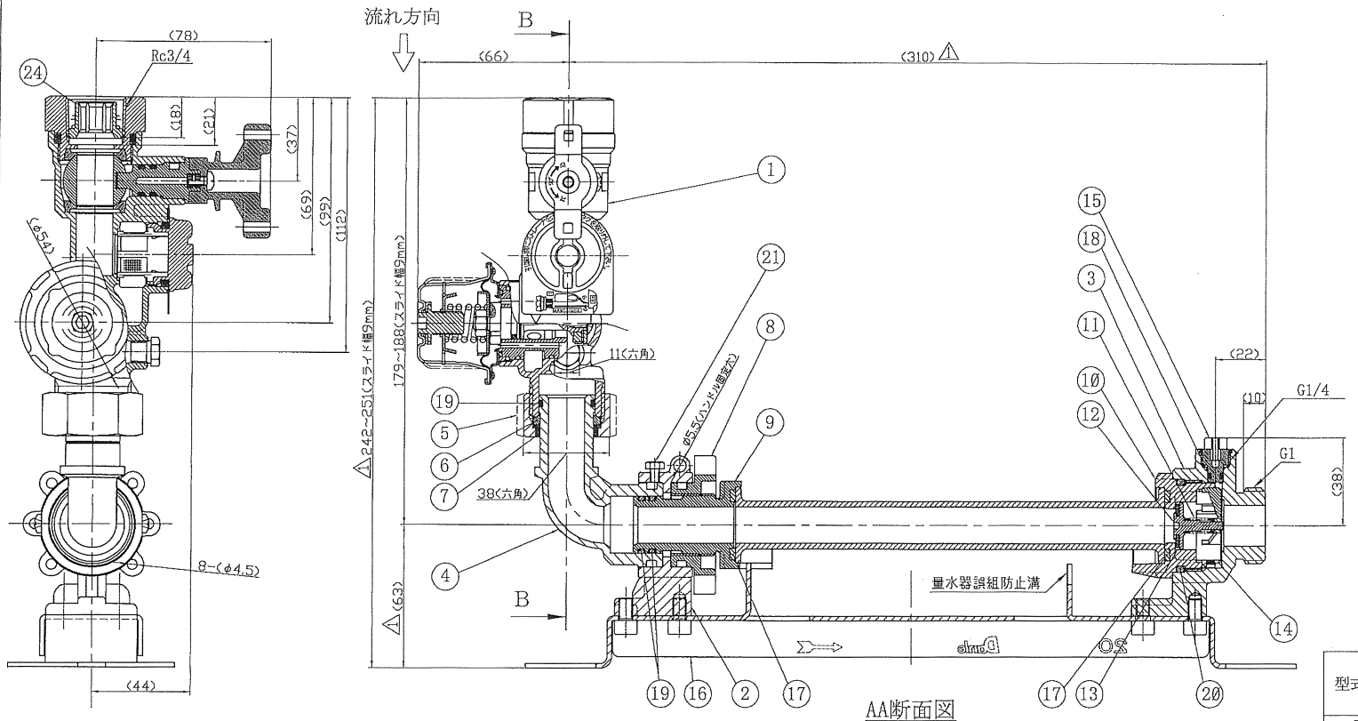
BB断面図
