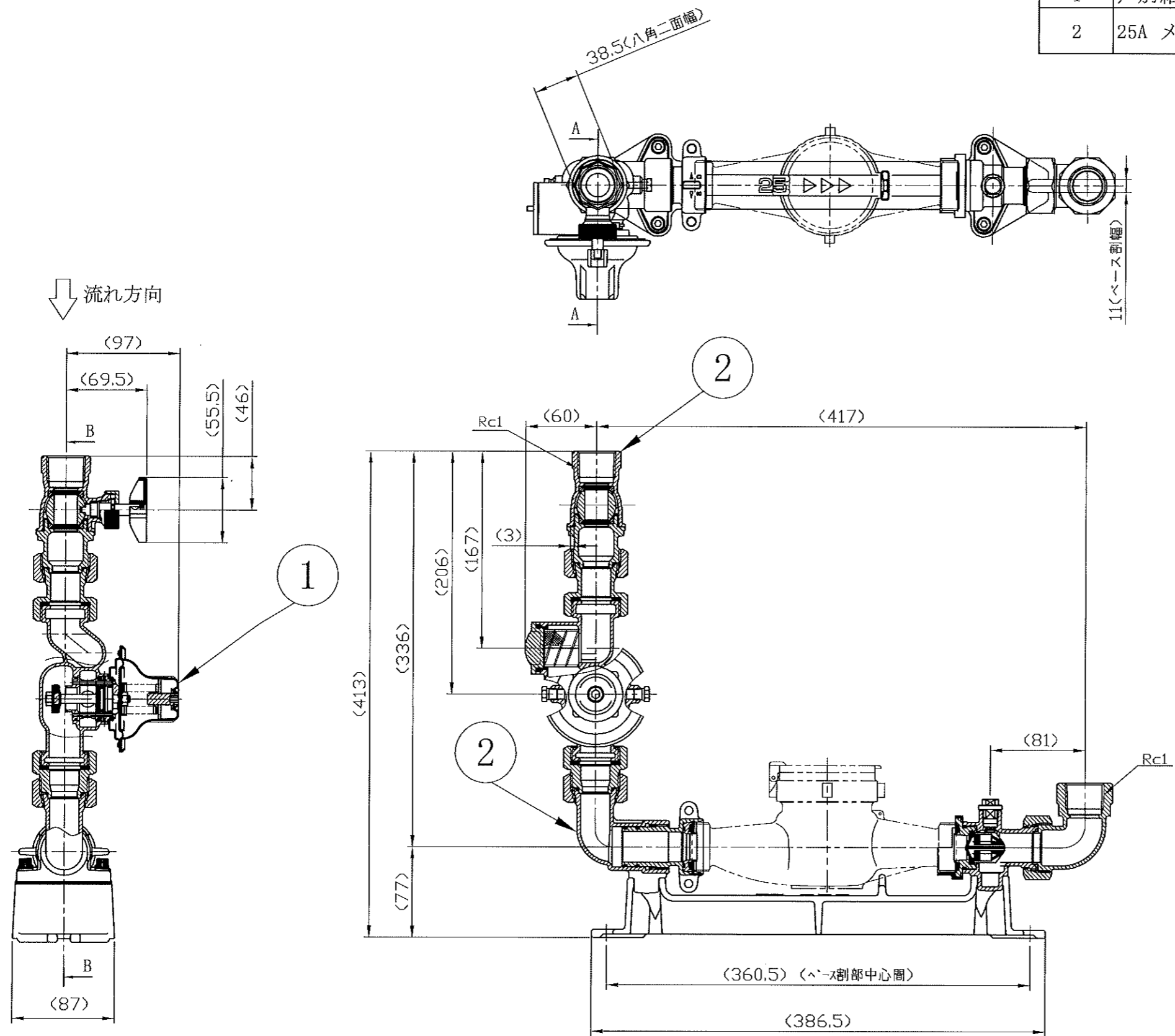
AA断面図
