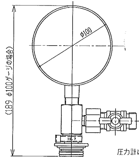
完成図(1/2)
