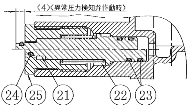
CC断面図 (部分) ※異常圧力検知弁部
