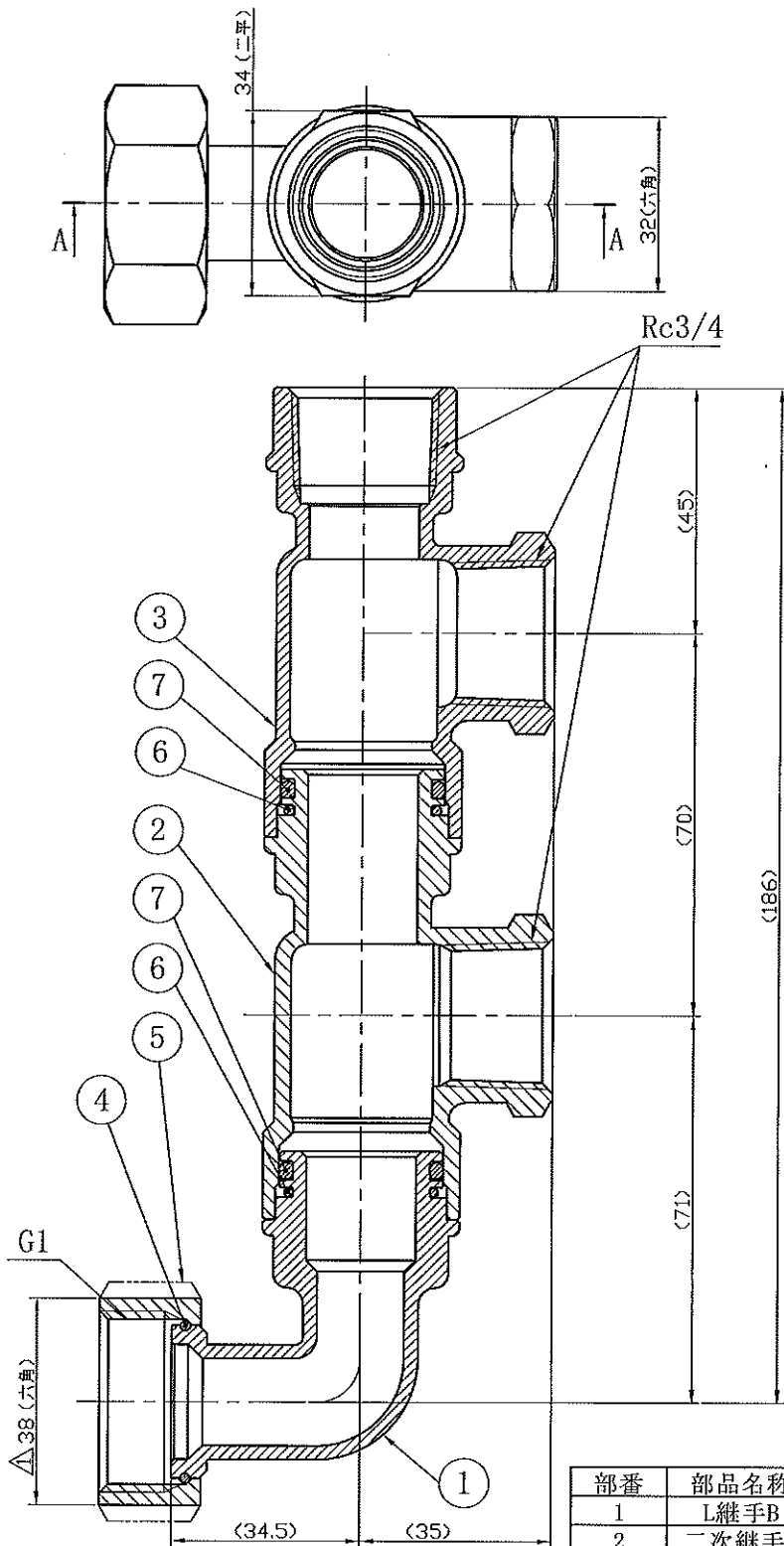
AA断面図
