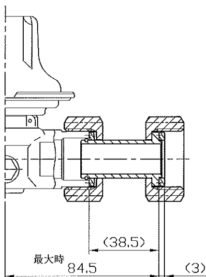
RU2034接続時(1:2)
