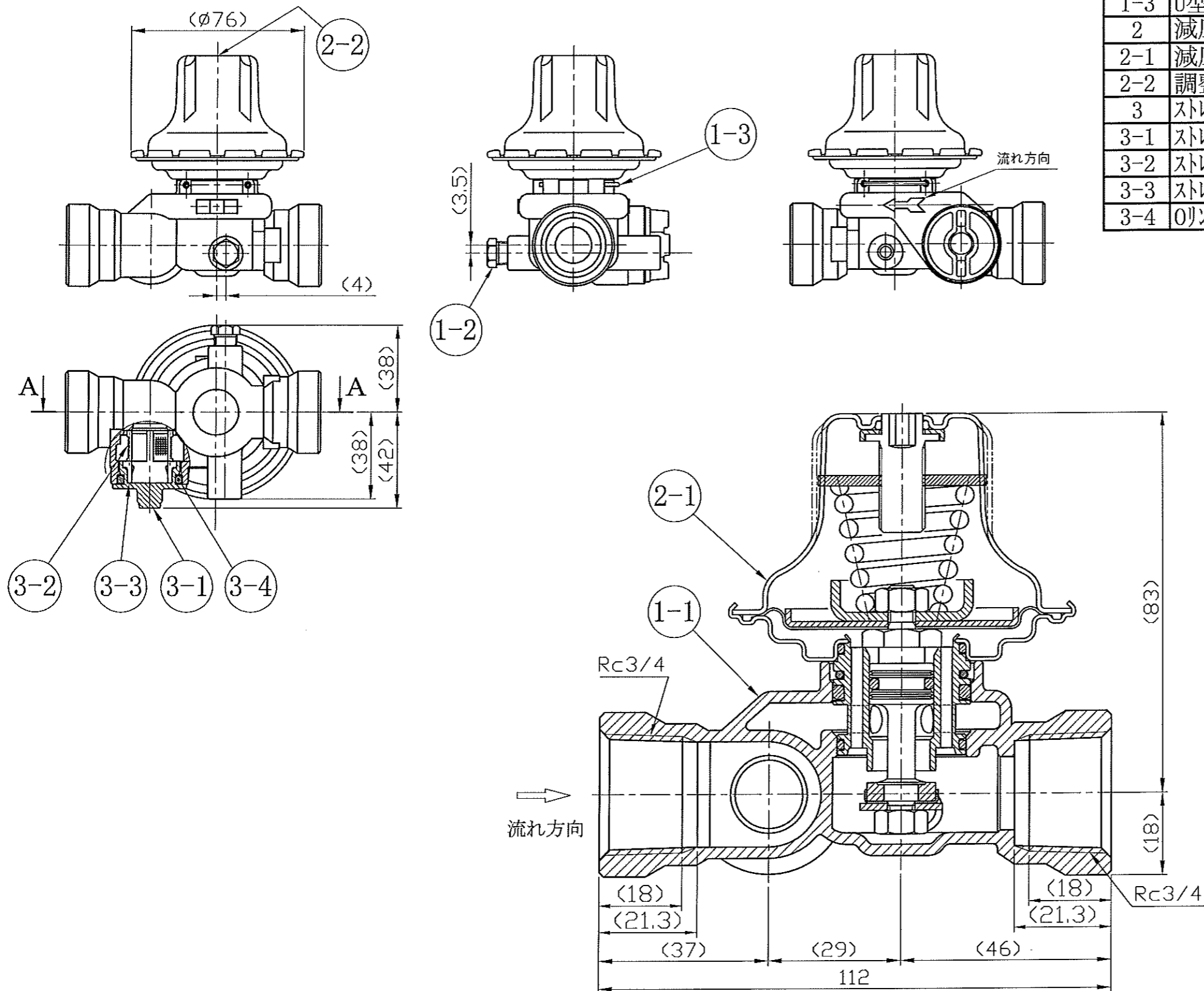
AA断面図(S=1:1)
